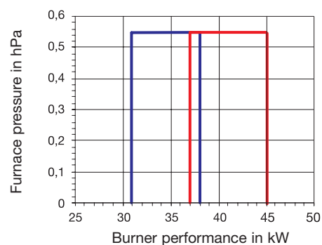
HL 60 NLV.2-S HL 60 PLV.2-S
